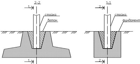
Рис. 1 Закрепление опор знаков в фундаменте
